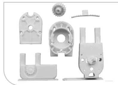
ITEM 63258 SET POLEA LATERAL COMPACTO PEL 1 DER
